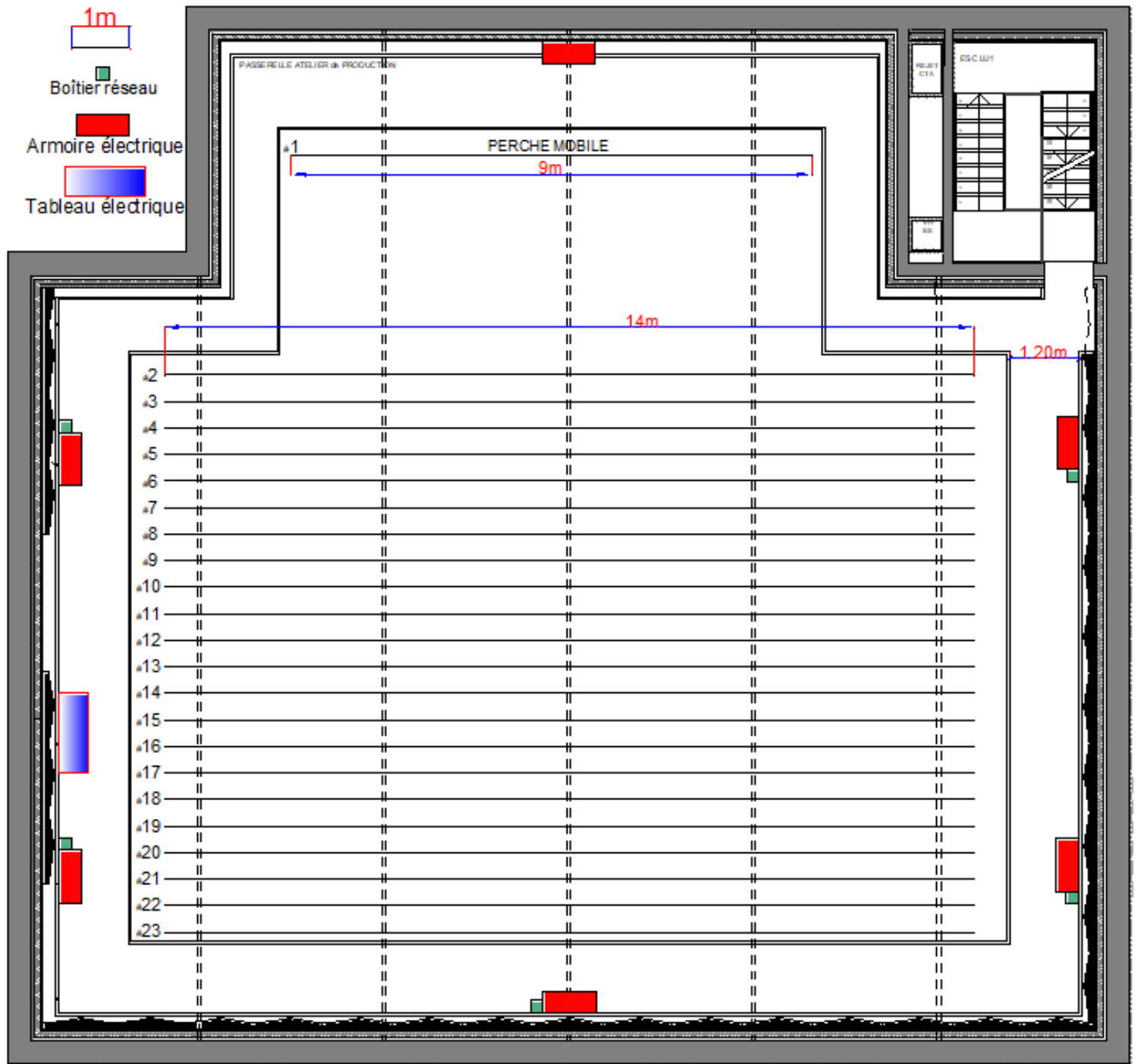
PLAN NIVEAU PASSERELLE
